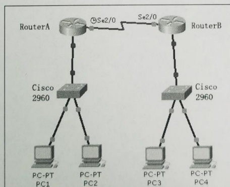
图 10-8 思考题 (1) 的实验拓扑图
