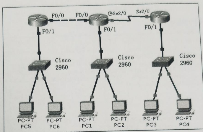
图 10-9 思考题（2）的实验拓扑图
