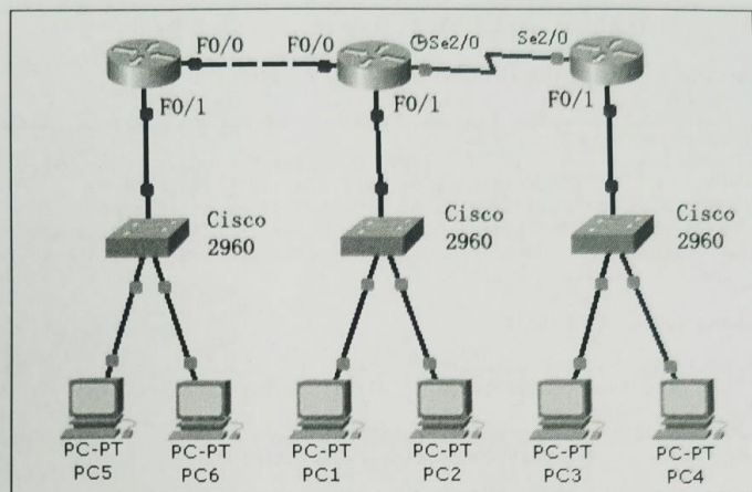
图 12-9 思考题（2）的拓扑图
