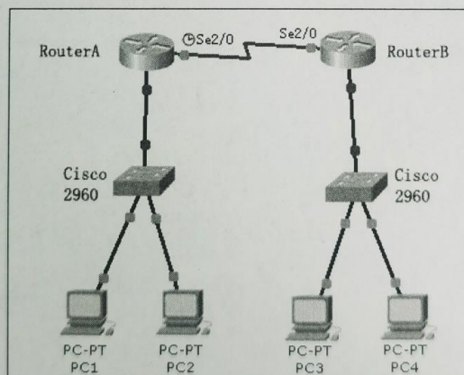
图 12-8 思考题 (1) 的拓扑图
