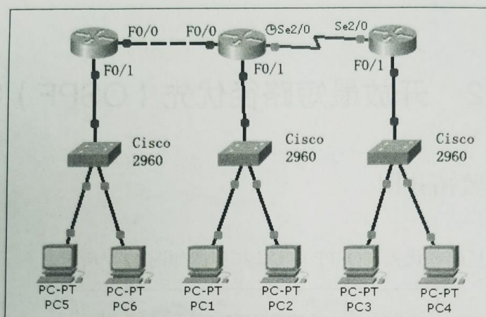
图 11-9 思考题 (2) 的拓扑图
