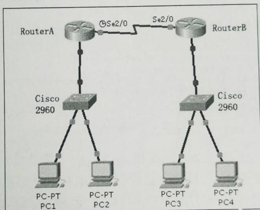
图 11-8 思考题 (1) 的拓扑图
